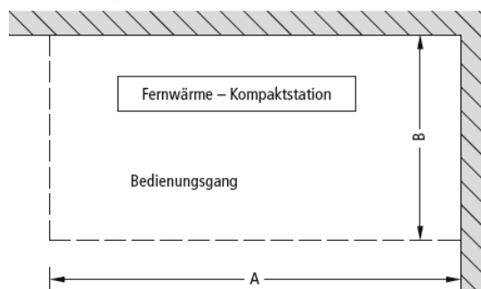
Platzbedarf Kompaktstation
