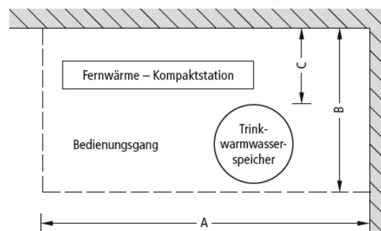
Platzbedarf Kompaktstation mit Warmwasserbereitung
